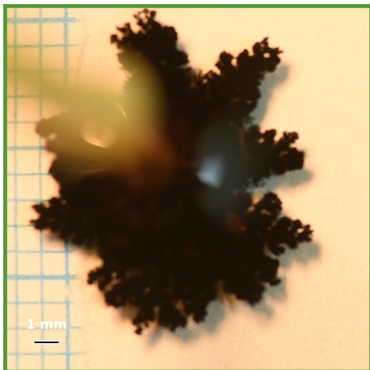
0.45 %* D = 1.93
