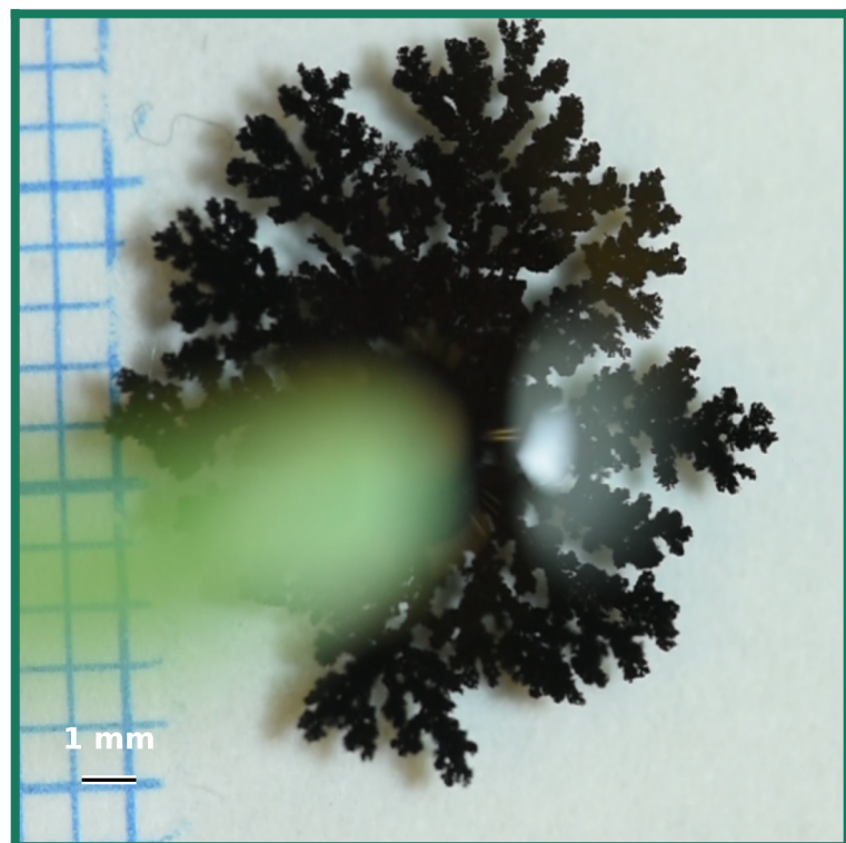
0.15 % D = 1.87
